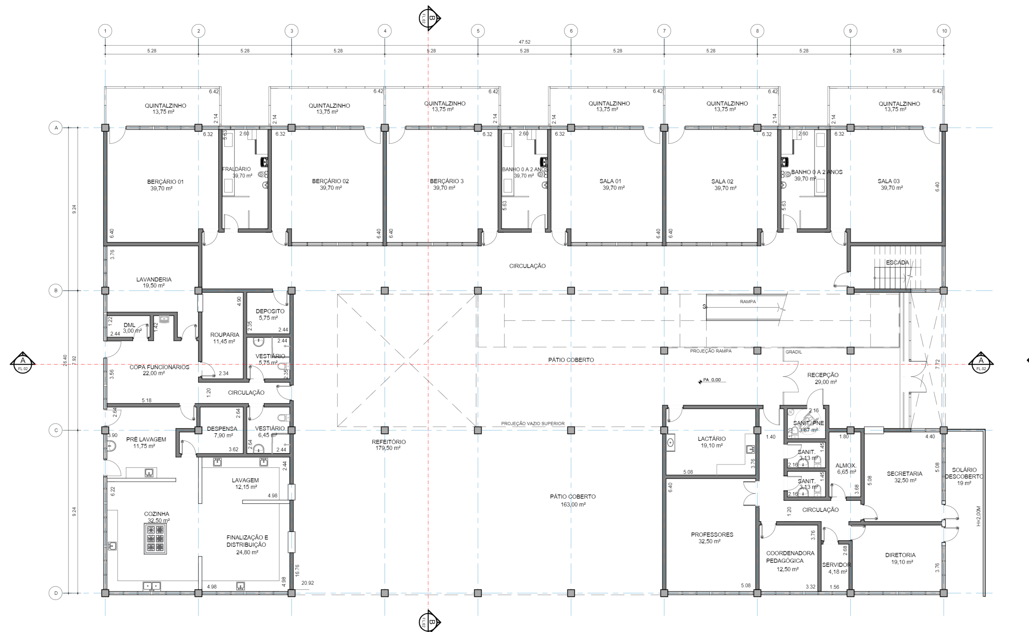
1 PAV. TÉRREO 1 : 100
