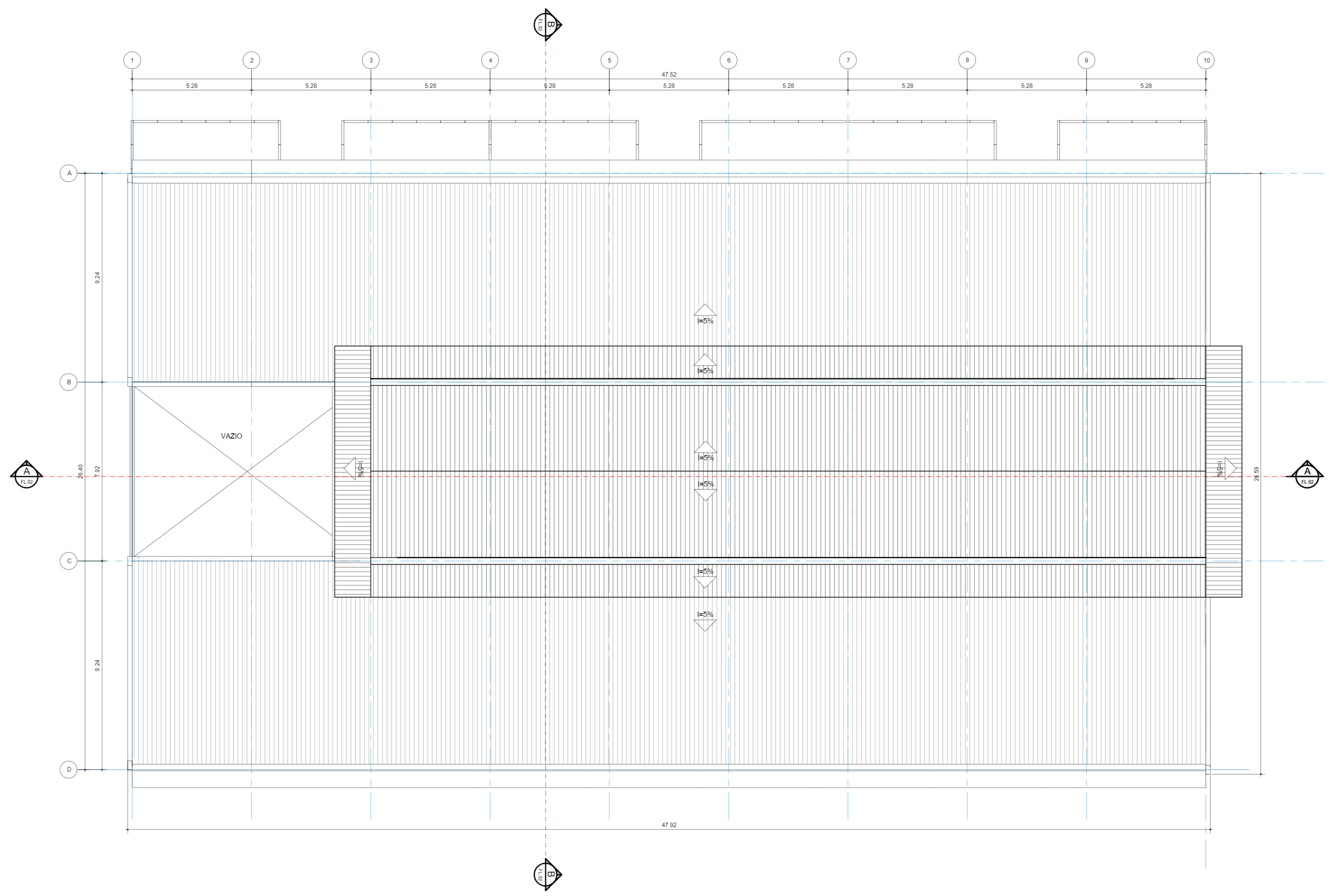
3 COBERTURA 1 : 100
