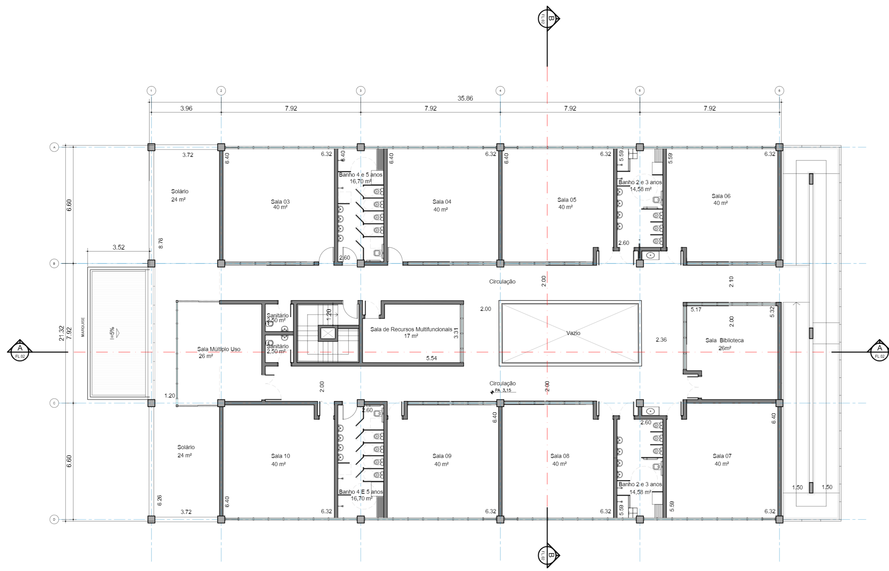
2 PAV. SUPERIOR 1 : 100
