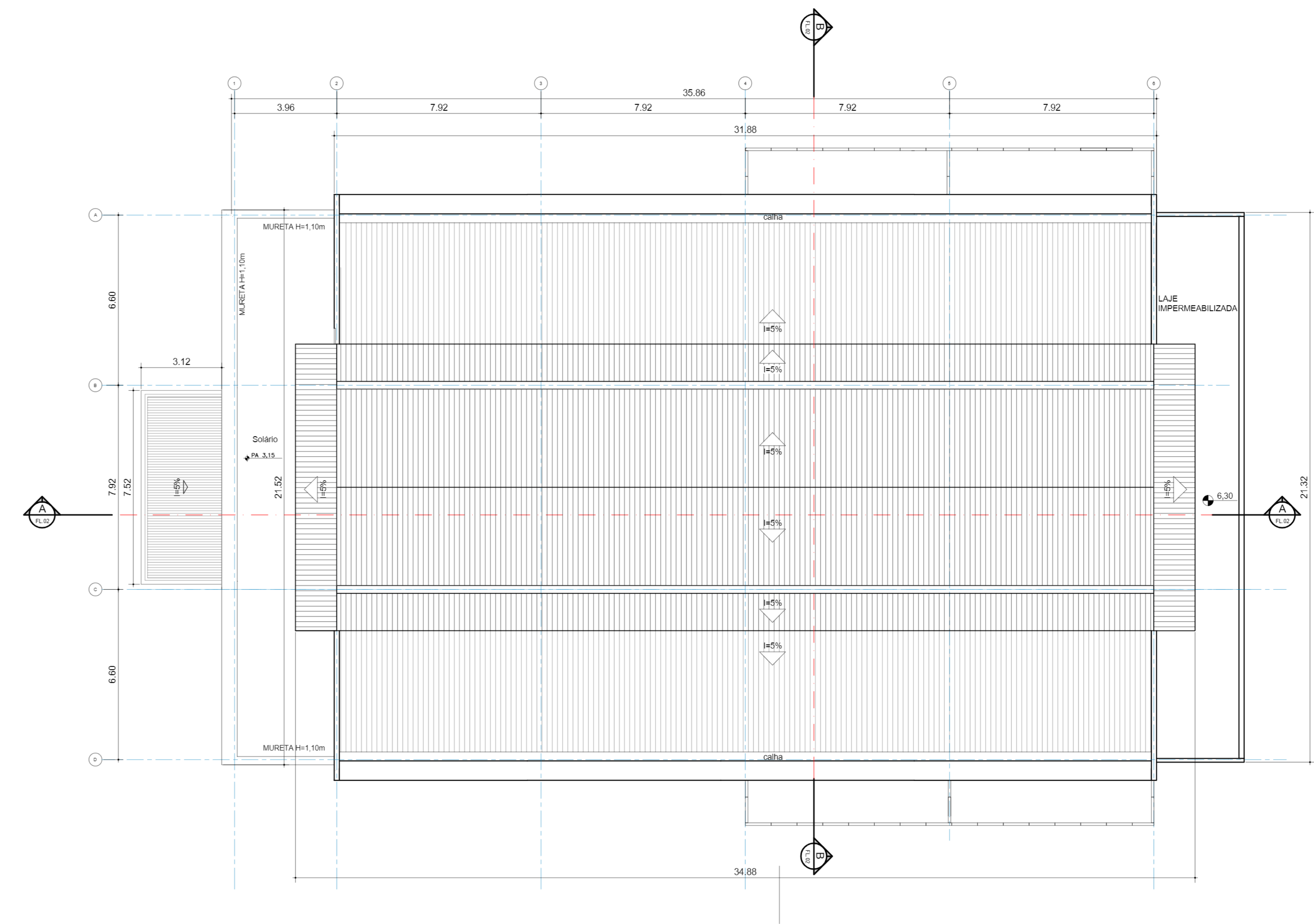
3 COBERTURA 1 : 100
